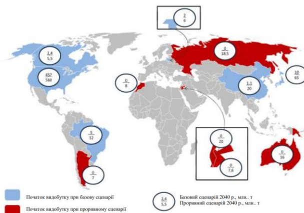
Рис. 3. Динаміка видобутку сланцевої нафти у 2040 р. у базовому сценарії та у сценарії "сланцевого прориву"
