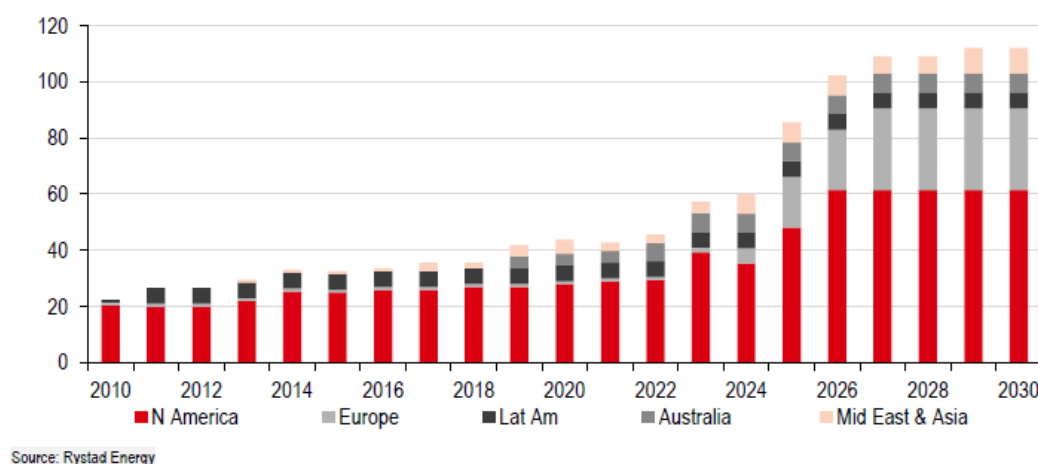
Рис. 2. Потужності технології CCS по країнам
