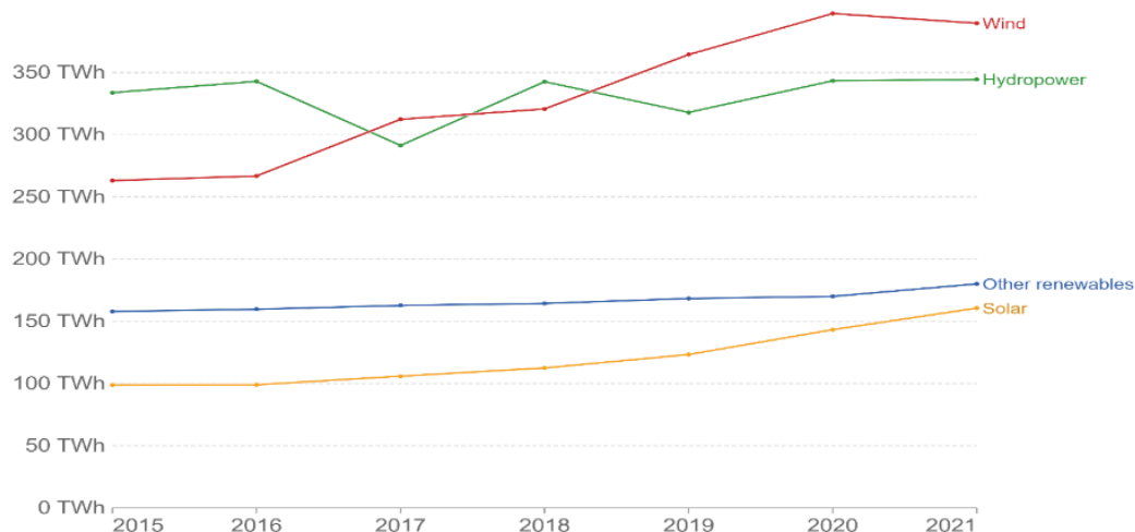
Рис. 1 – Використання ВДЕ в ТВт-год країнами ЄС, 2015-2021 рр.
