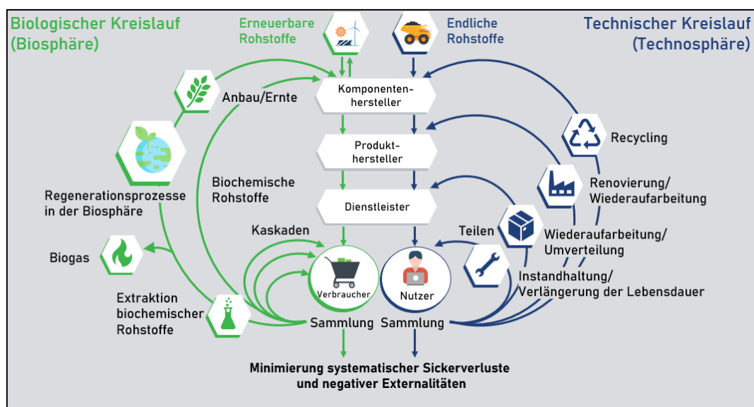
Abbildung 1. Schema der Kreislaufwirtschaft [1]
