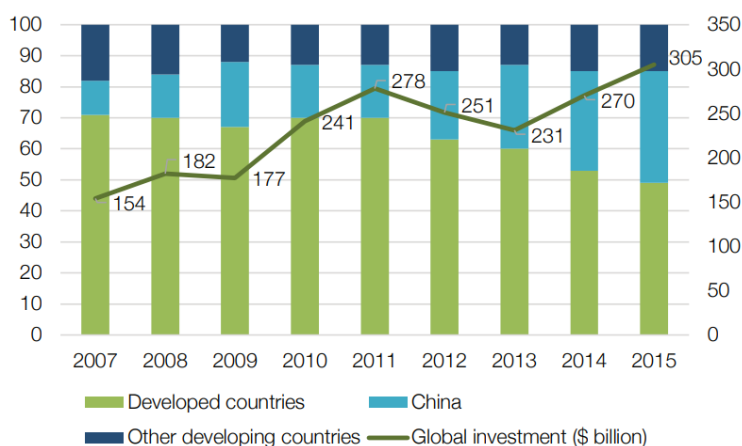
Рис. 2. Світові інвестиції у розвиток відновлюваної енергетики
