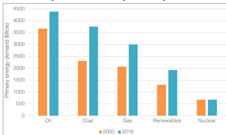
Рис. 1. Світовий попит на первинну енергію за джерелами енергії (нафта, вугілля, газ, відновлювані джерела енергії, атомна енергетика)
